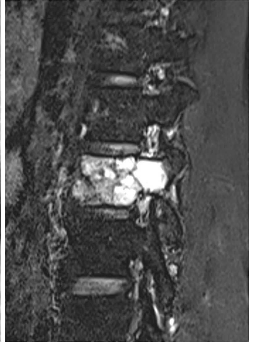
FST2WI
