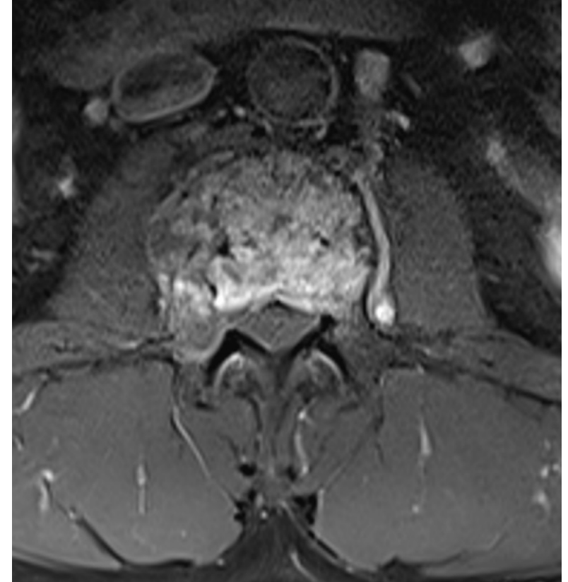
GdFST1WI
