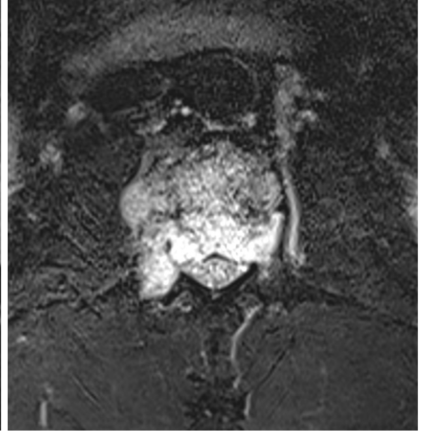
FST2WI
