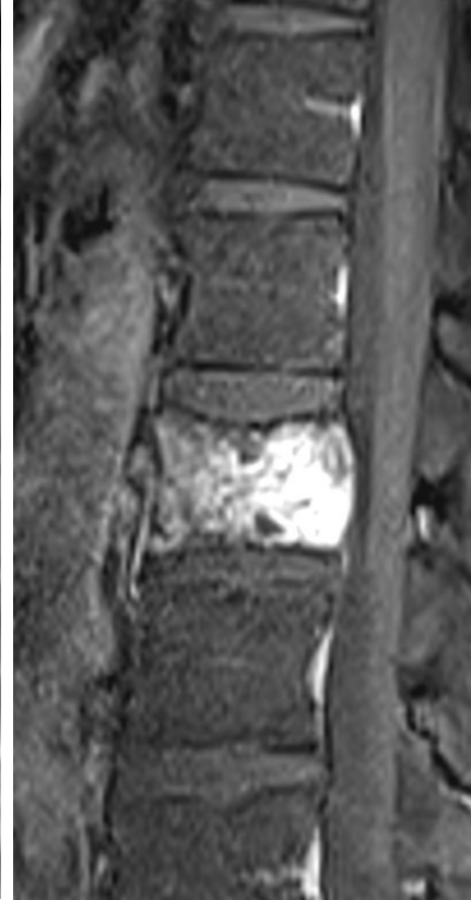
GdFST1WI
